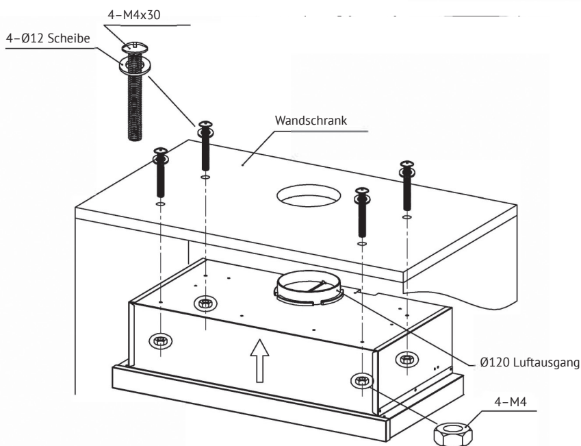
Aufstellungsplan
