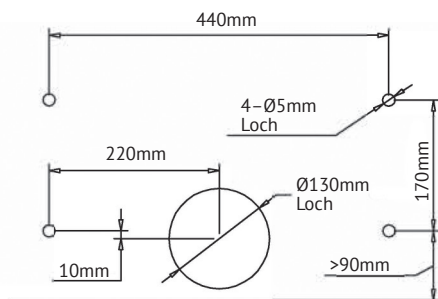
Bohrbild
